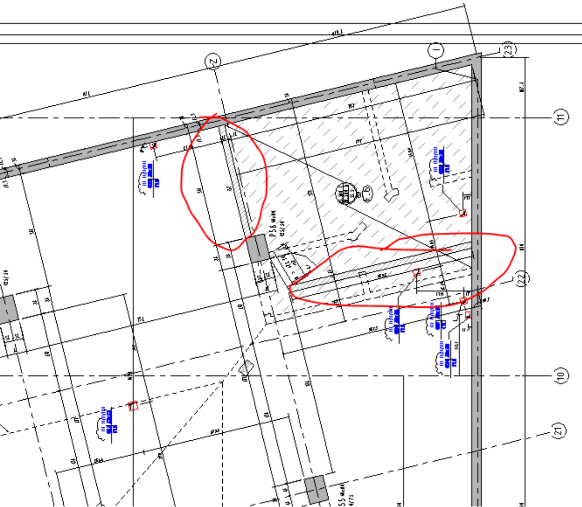
MOTIF HACHURE MUR MACONNERIE DANS LA VUE TOURNE DE 90° DANS LA FEUILLE
